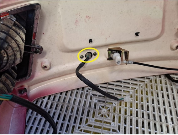
Irrota kilven valon kiinnitysruuvit. (ristipäämeisseli ph2).
